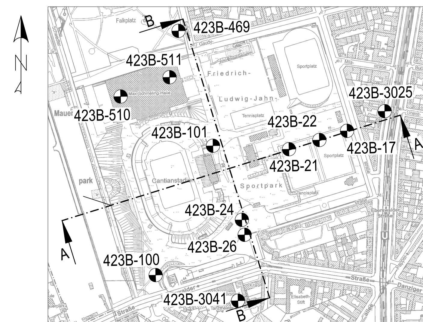
Übersichtsplan; M 1:5.000
