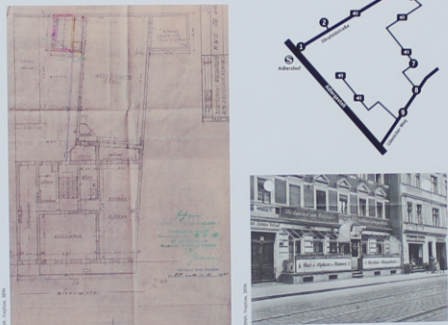
Raucherhaus (Raucherhaus), Saalplan im Restaurant Ratskeller, 1940 Construction drawing (Saal), Hall complex in the Ratskeller restaurant, 1940 Raucherhaus (Raucherhaus), Saalplan im Restaurant Ratskeller, 1940 Construction drawing (Saal), Hall complex in the Ratskeller restaurant, 1940
