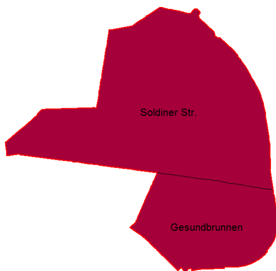
Abb. 17: Umweltgerechtigkeit
