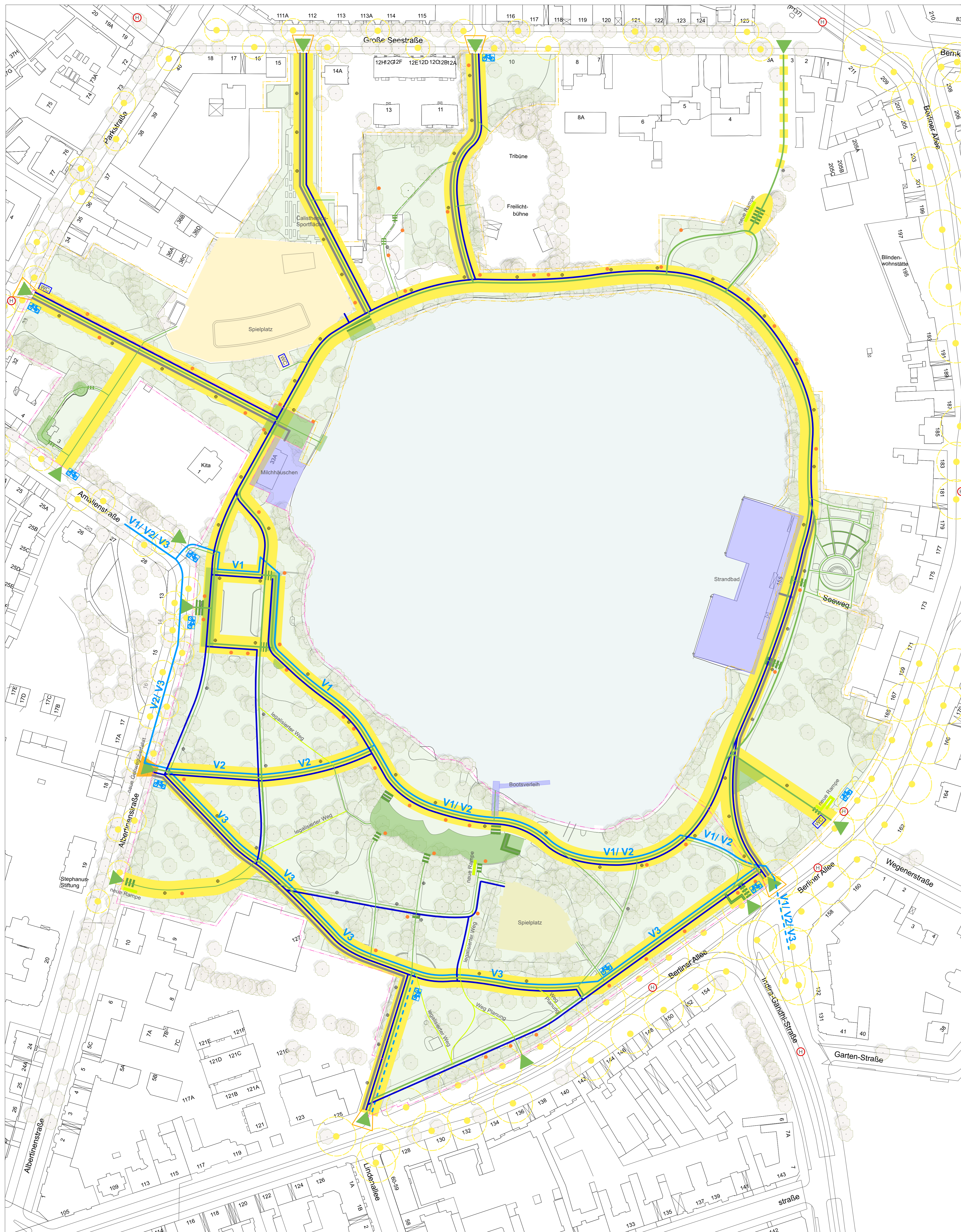
Entwurf: Wegekonzept M 1:1000
