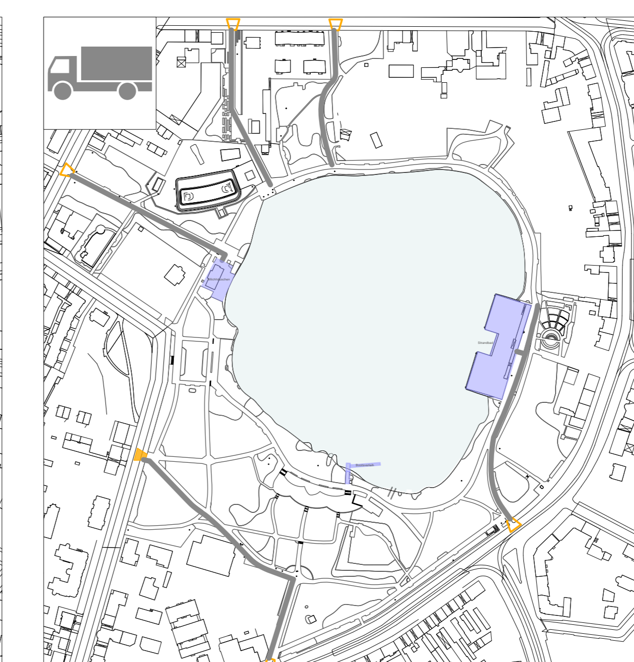
befahrbarer Weg bis 16 t - z.B. für Anlieferung
